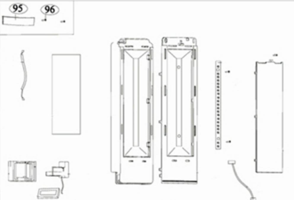
120 Fridge airflow assembly ASSIEME ILLUMINAZIONE AIRFLOW FRIGORIFERO
